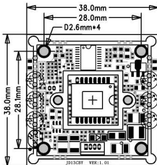
Рис.2. Установочные размеры.
